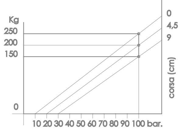
DIAGRAMMA SPINTE
